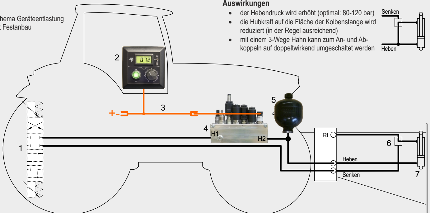
1 Traktor Steuergerät, 2 Bediengerät, 3 Kabelsatz, 4 Entlastungsblock, 5 Druckspeicher, 6 3-Wege Hahn, 7 Hubzylinder
