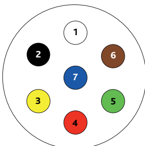
Ansicht Stecker
