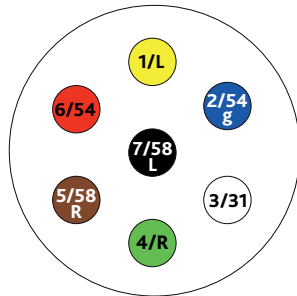
Ansicht Kabelseitig
