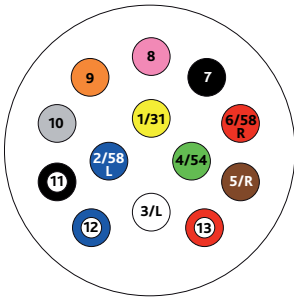
Ansicht Stecker
