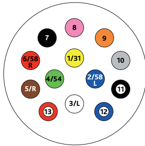
Ansicht Kabelseitig
