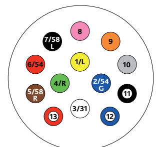
Ansicht Kabelseitig
