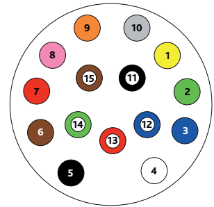
Ansicht Kabelseitig
